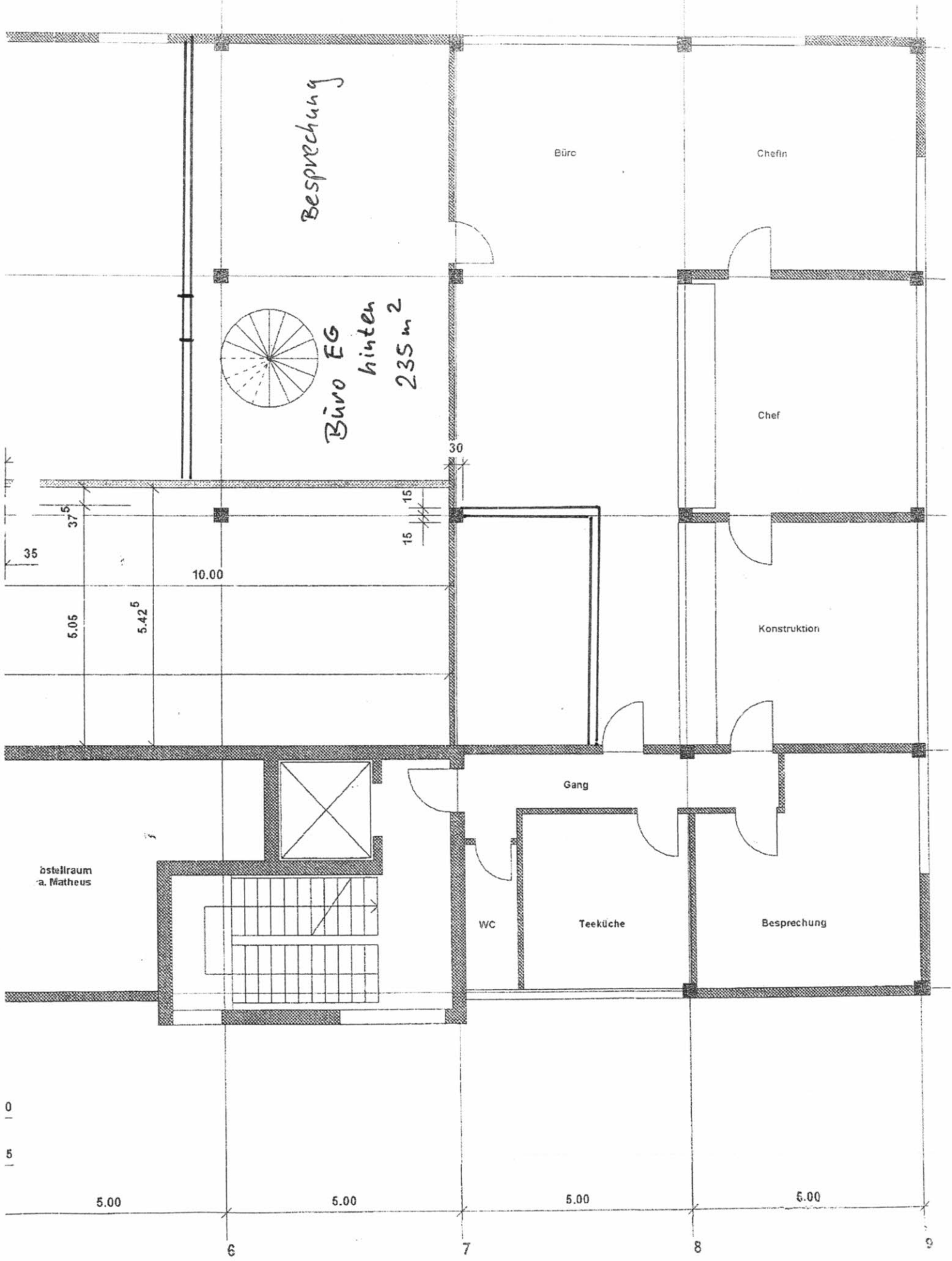
Anlage 1: Büro- und Sozialräume EG
